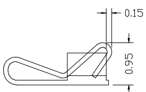
极限压下高度
